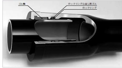
■ NS 形 呼び径300~450
