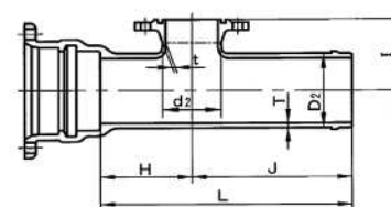
浅埋設用フランジ付T字管
