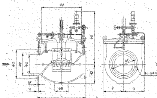
呼び径：350～400mm
