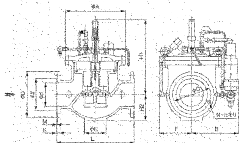
呼び径：350～400mm
