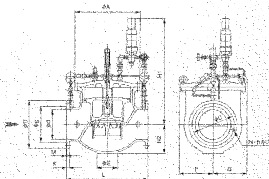
呼び径：250～300mm
