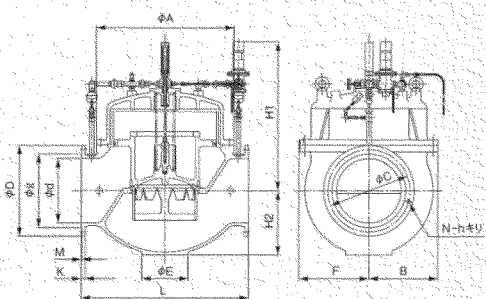
呼び径：450～800mm
