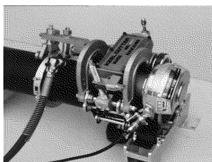
切断機(小型)
