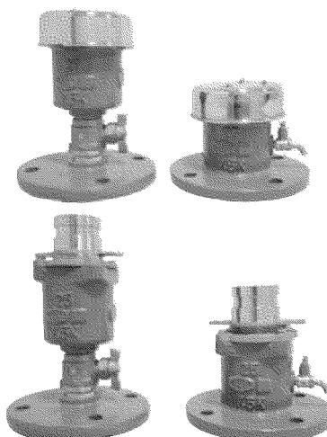
(口金付(オプション)取付状況)
